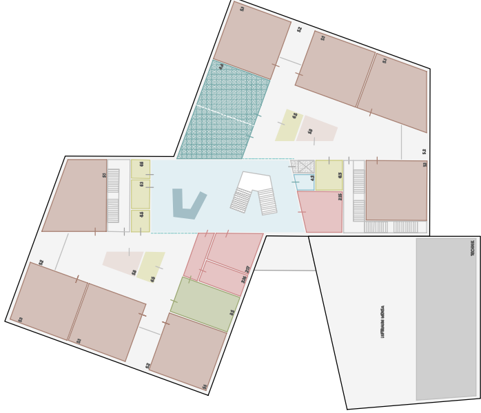
1. Obergeschoss
